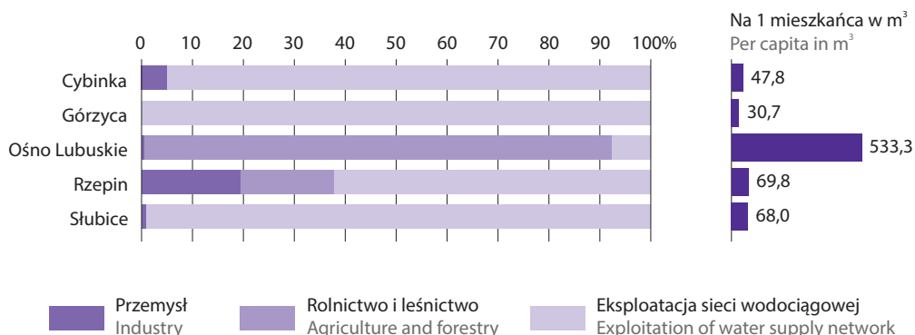
Wykres 93. Zużycie wody na potrzeby gospodarki narodowej i ludności w 2022 r. Chart 93. Water consumption for needs of the national economy and population in 2022
