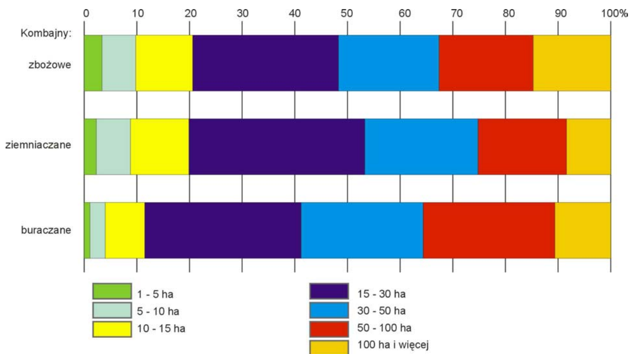
Wykres 8. Struktura kombajnów użytkowanych w indywidualnych gospodarstwach rolnych według grup obszarowych UR w 2002 r.
